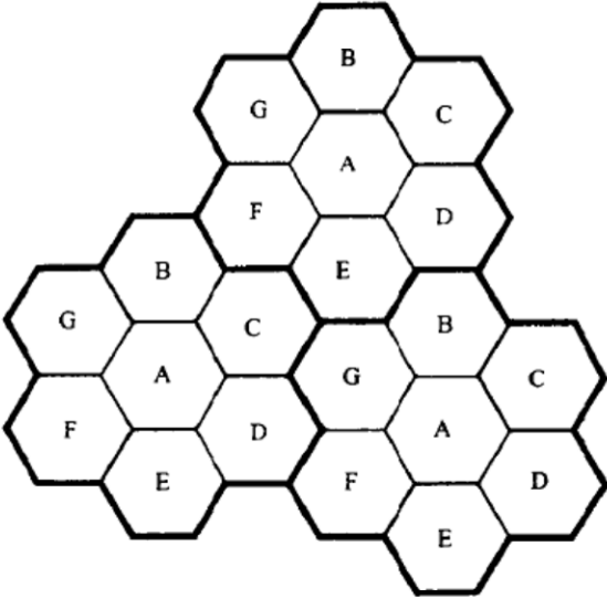
Fig 2.1: Frequency reuse( N=7)
